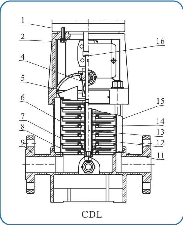
截面图 CDL,CDLF1,2,3,4
