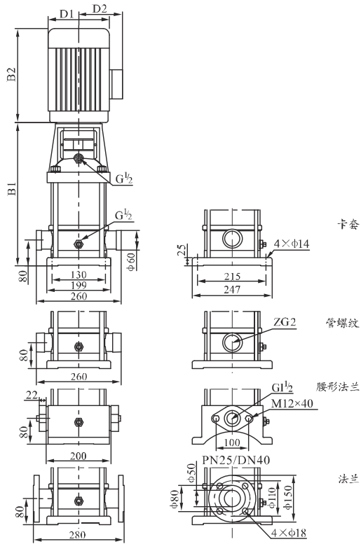
安装图
