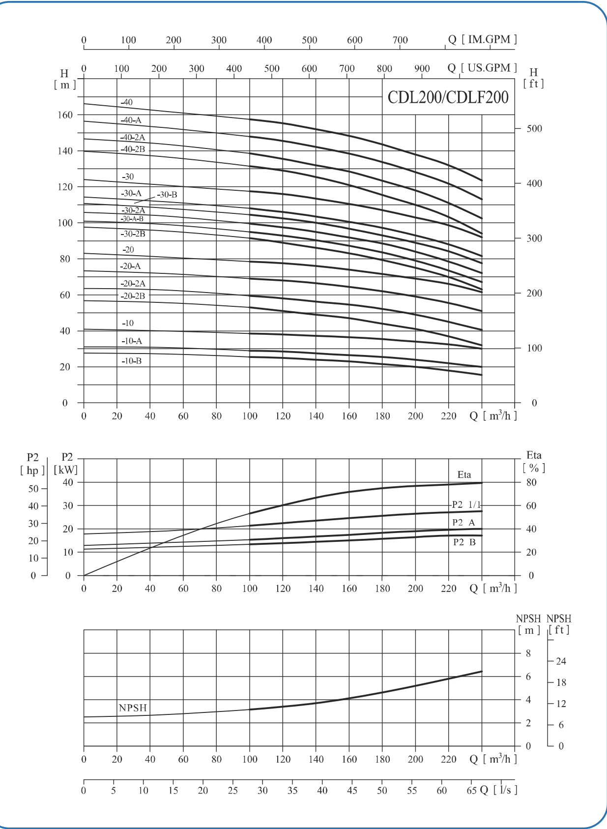
性能曲线
