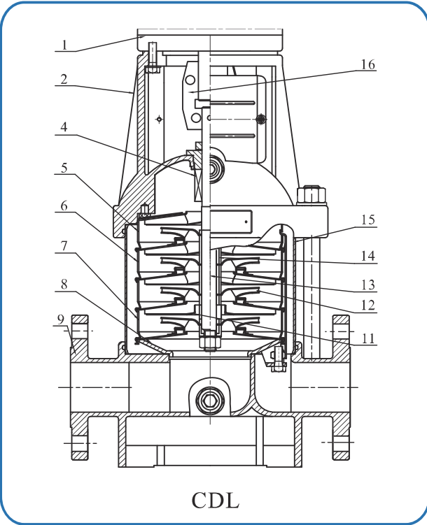
截面图 CDL,CDLF8,10,12,15,20
