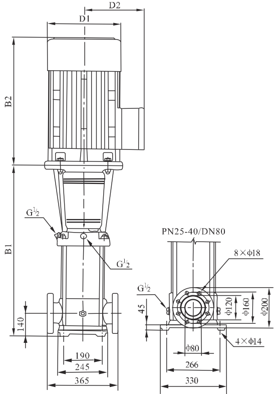
安装图
