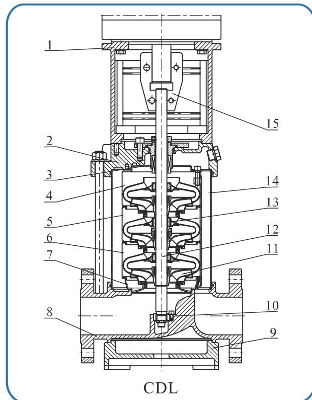
截面图 CDL,CDLF32,42,65,85
