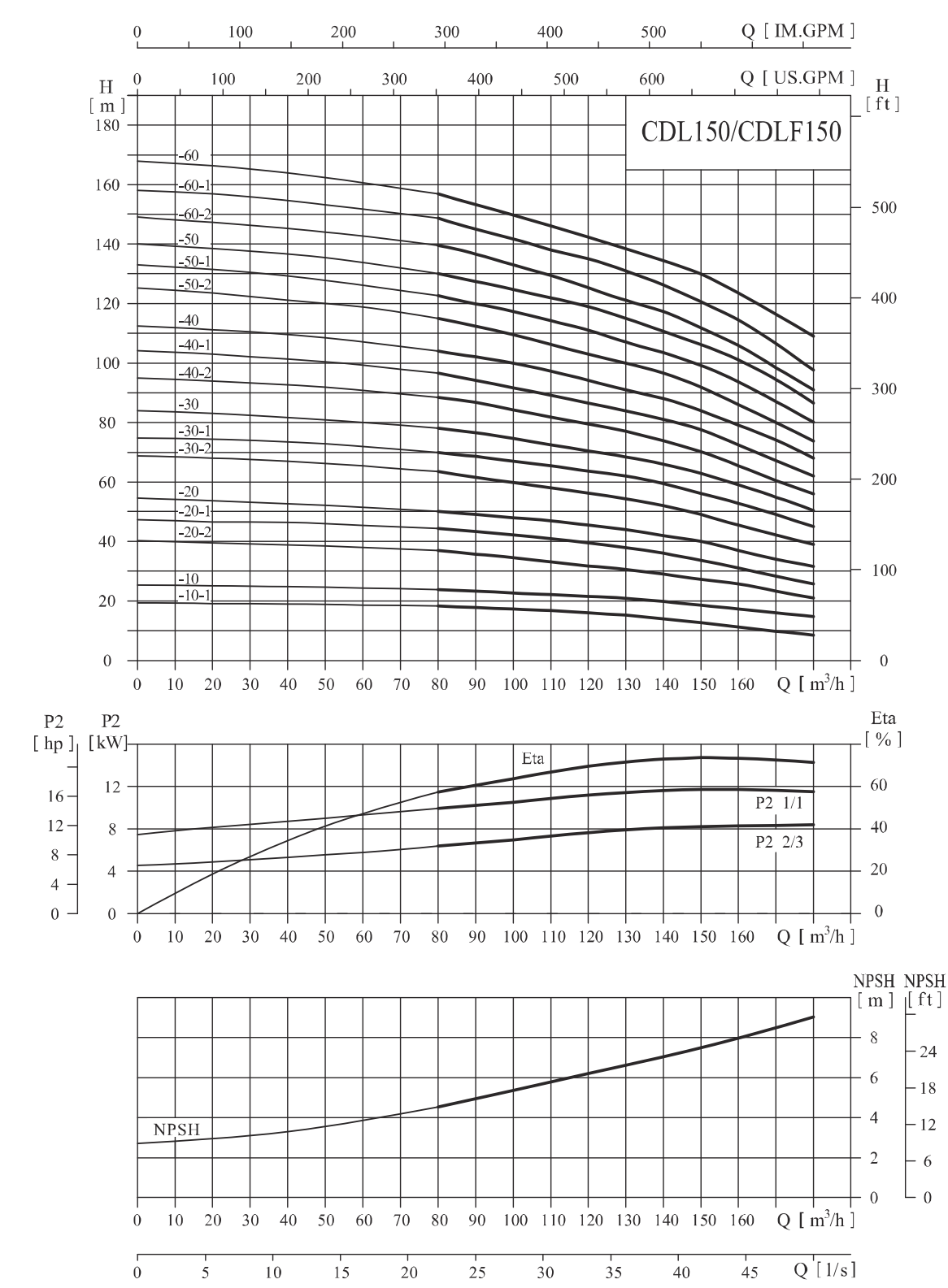
性能曲线
