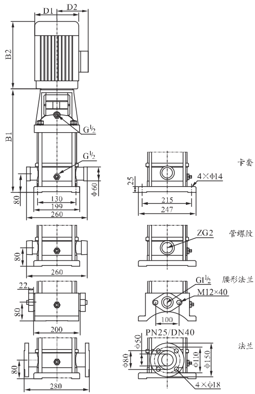
安装图
