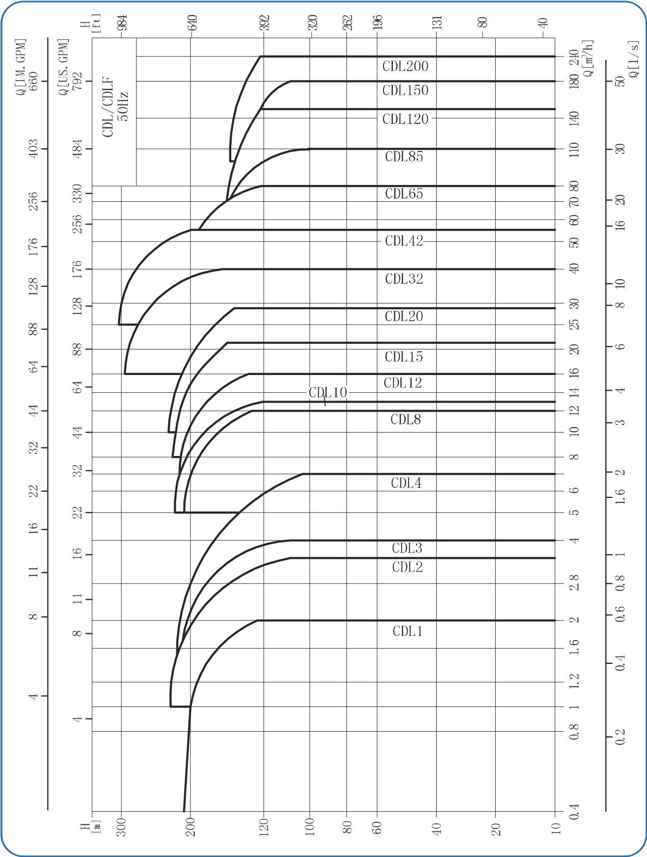
性能范围
