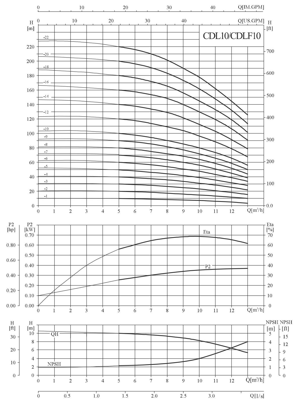
性能曲线
