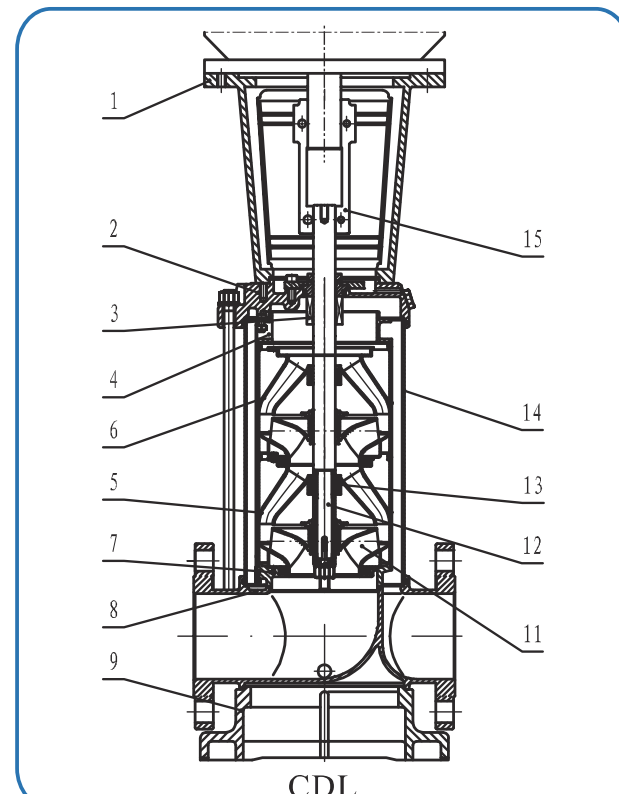
截面图 CDL,CDLF120,150,200
