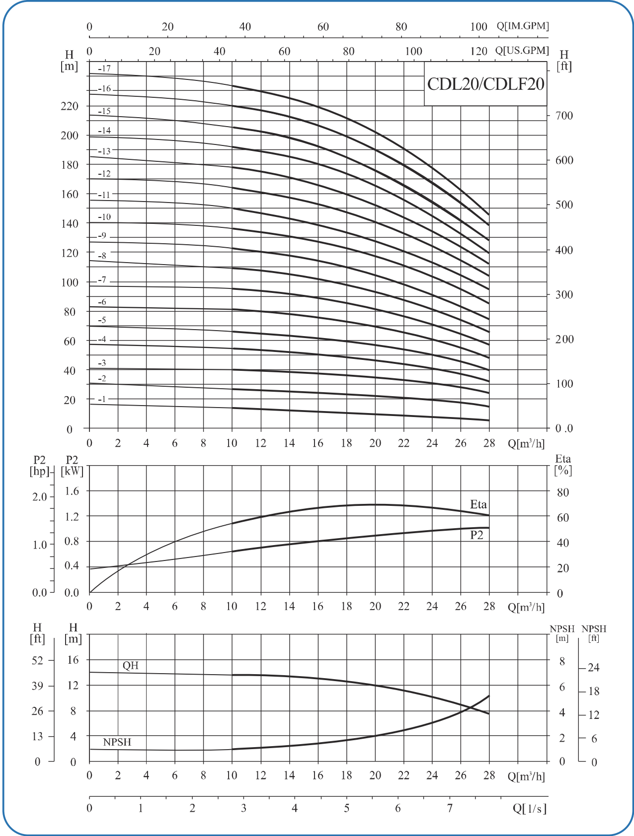
性能曲线
