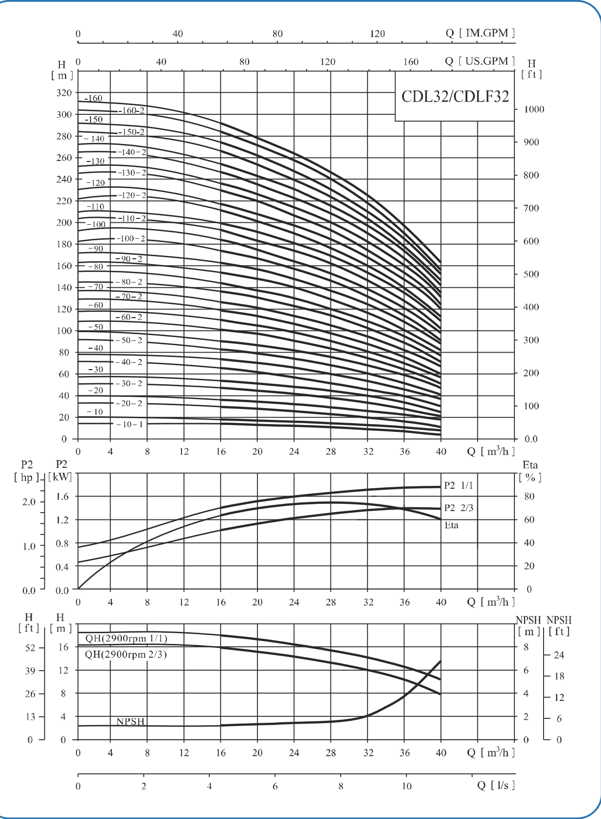
性能曲线
