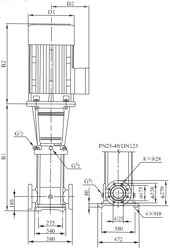
安装图
