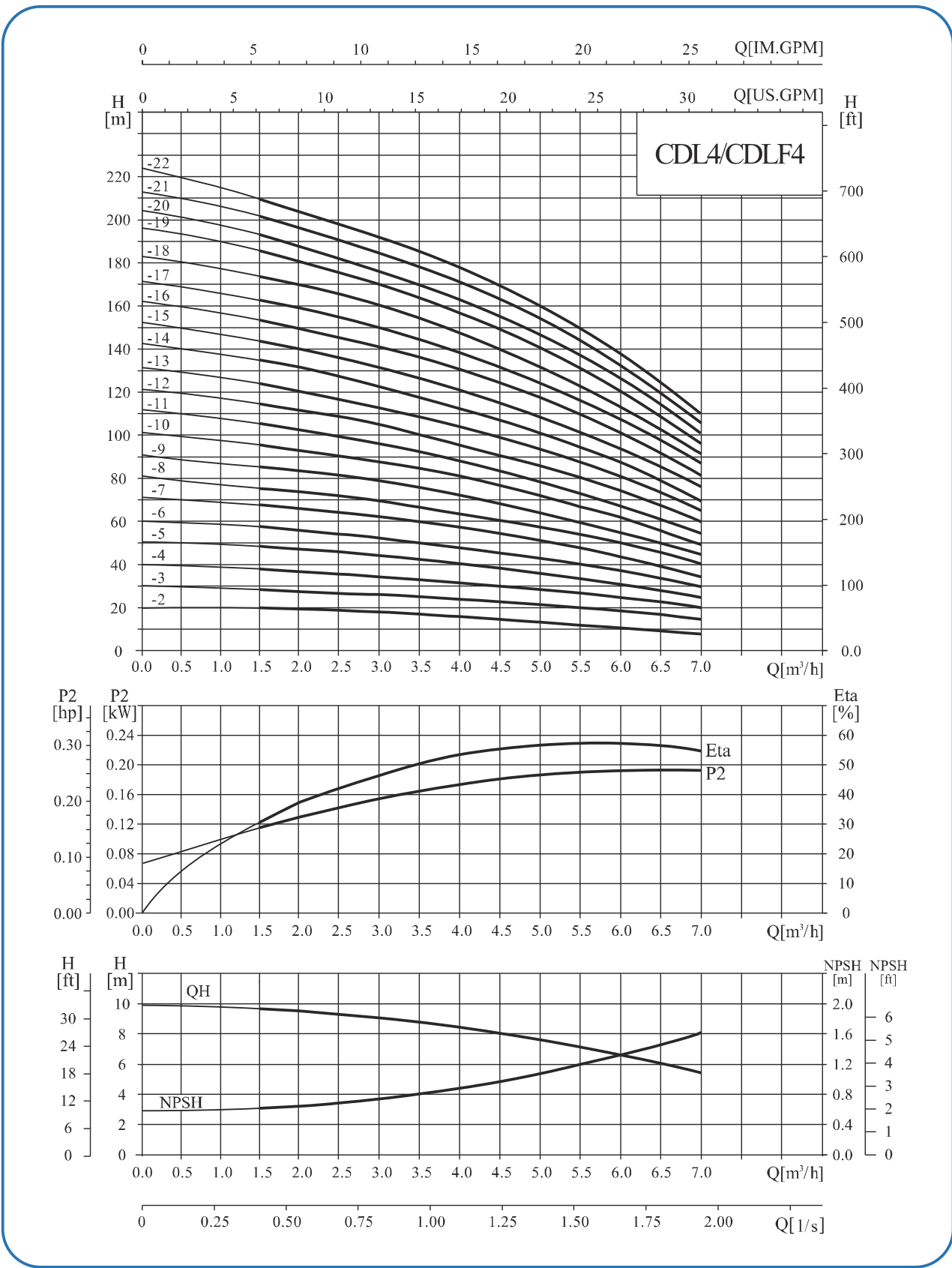
性能曲线
