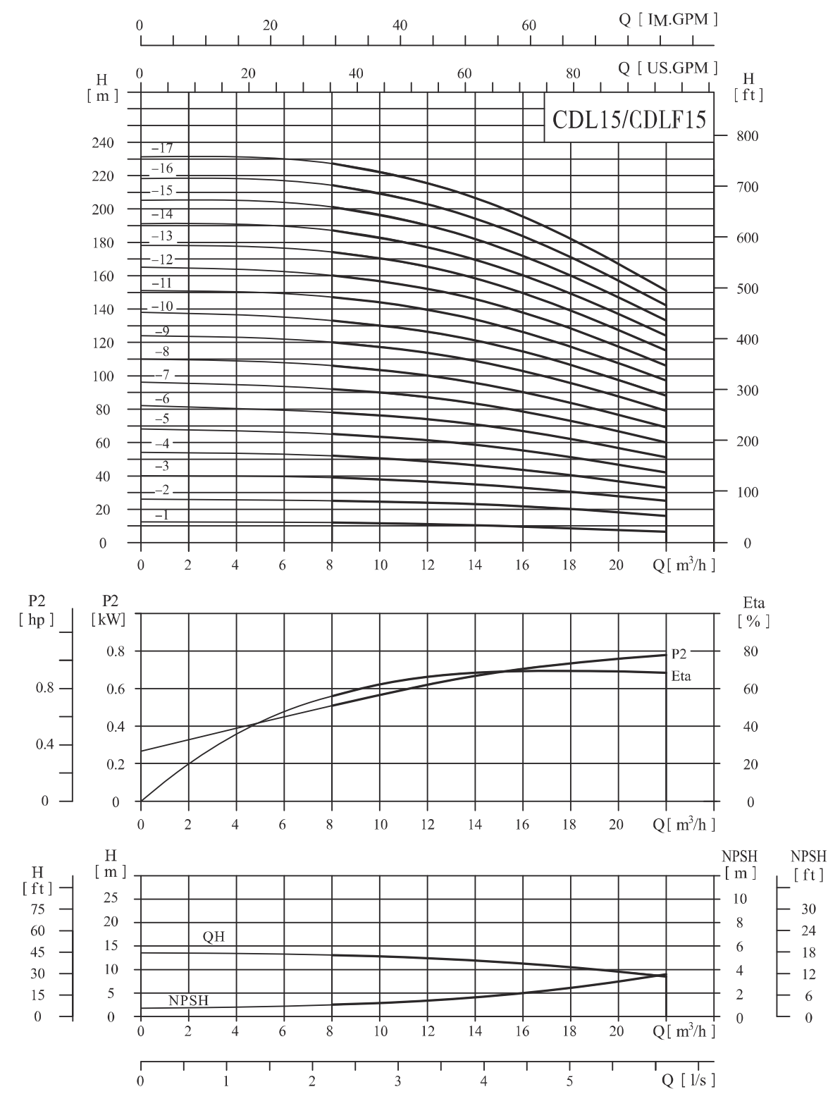
性能曲线
